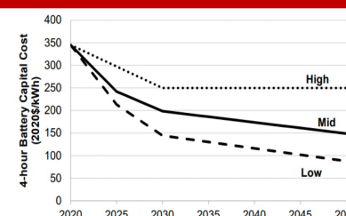
锂电池储能成本趋势
