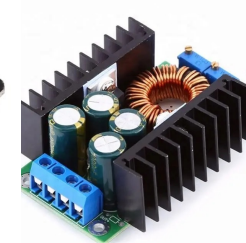
电源模组
