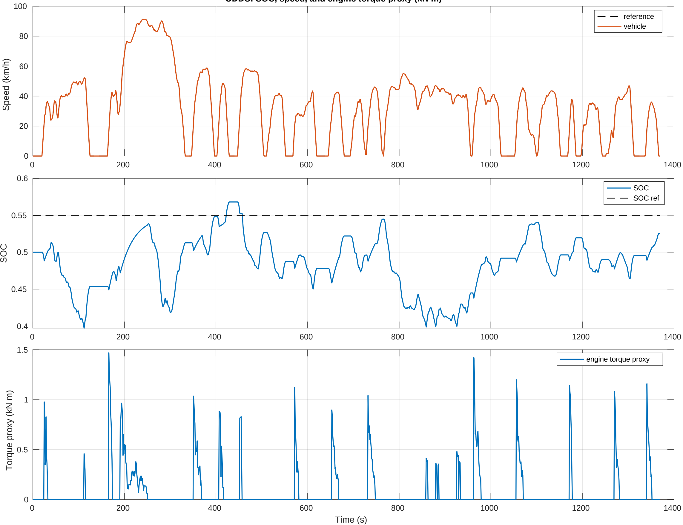
UDDS: SOC, speed, and engine torque proxy (kN m)
