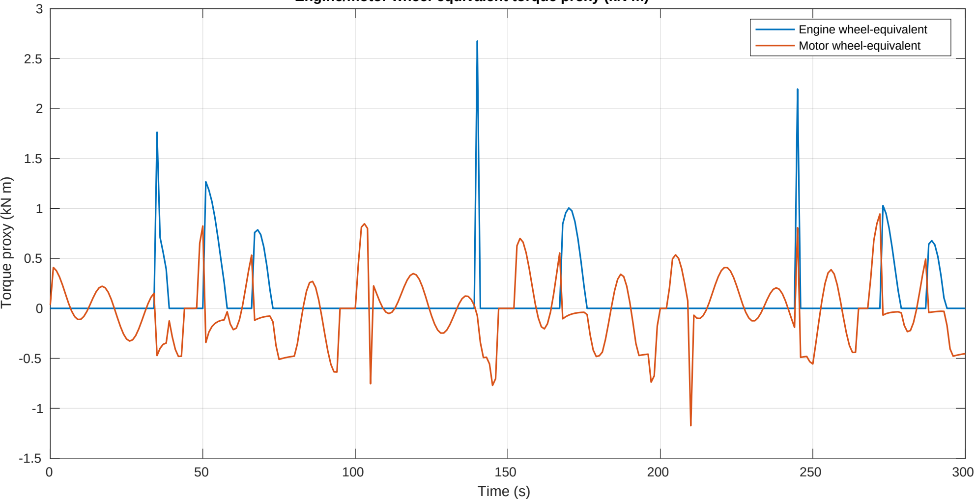
Engine/motor wheel-equivalent torque proxy (kN m)
