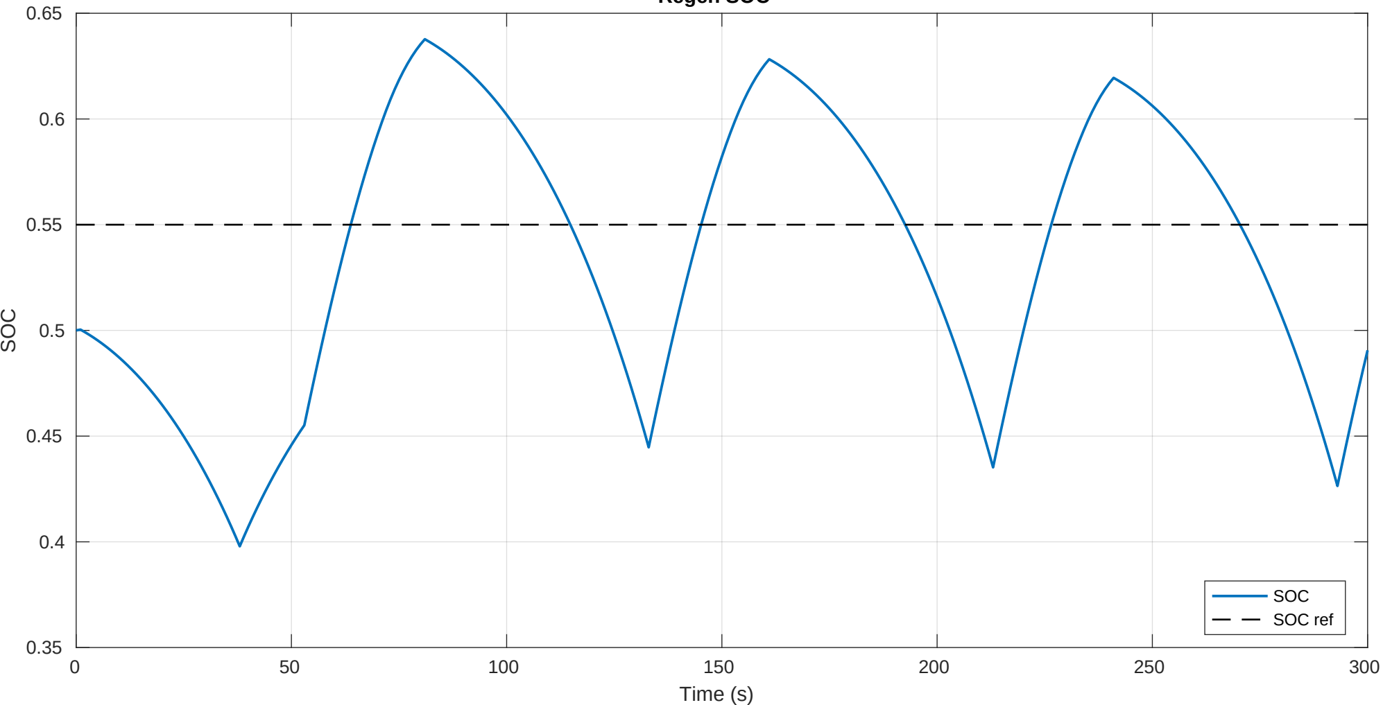
Regen SOC
