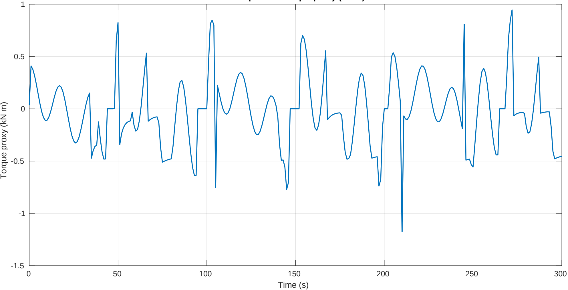
Motor wheel-equivalent torque proxy (kN m)
