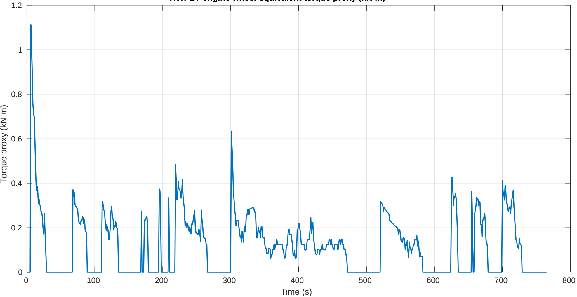
HWFET engine wheel-equivalent torque proxy (kN m)
