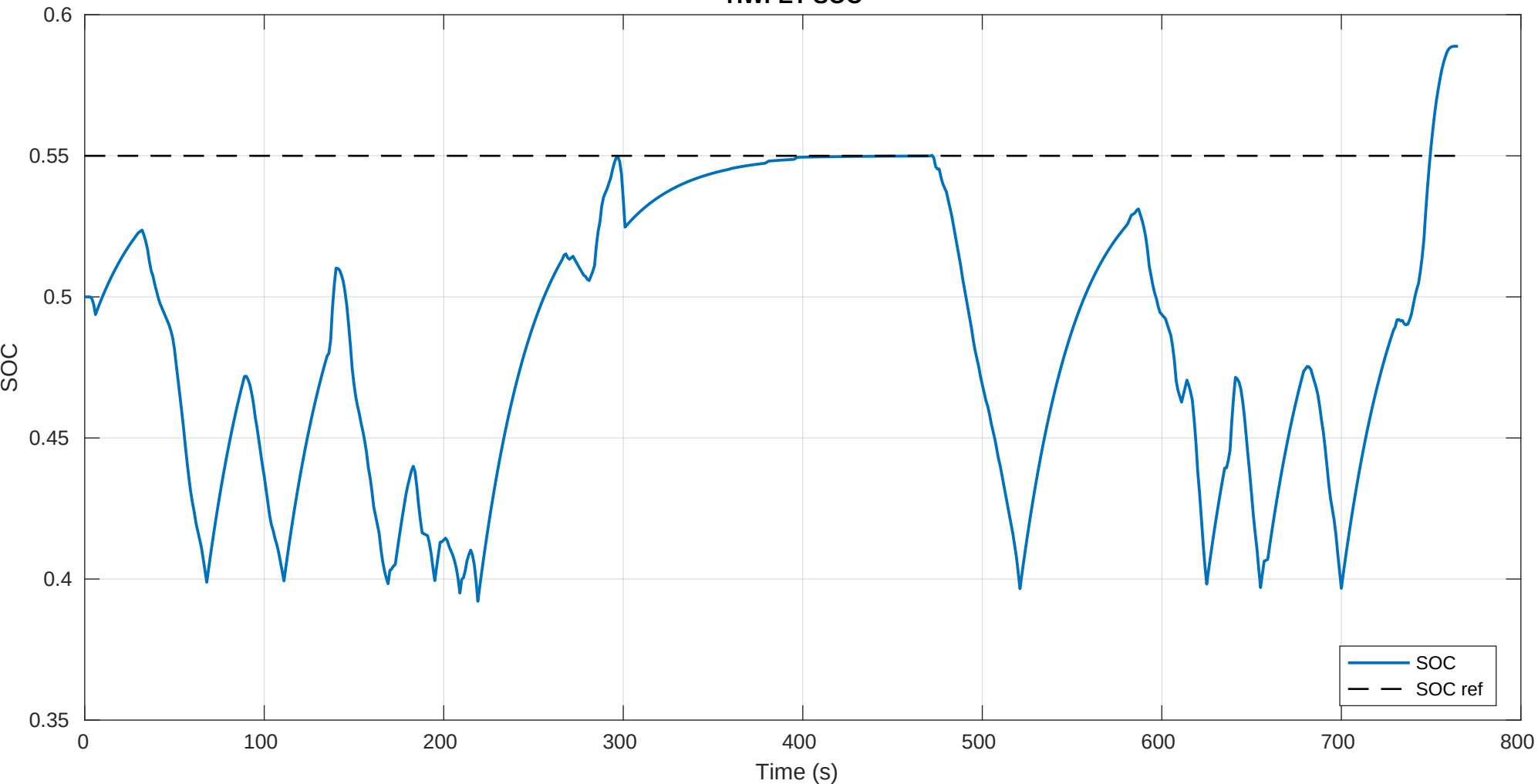
HWFET SOC
