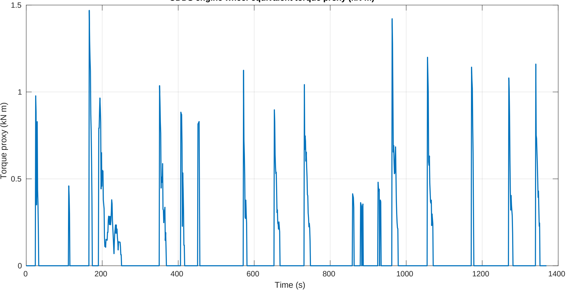
UDDS engine wheel-equivalent torque proxy (kN m)
