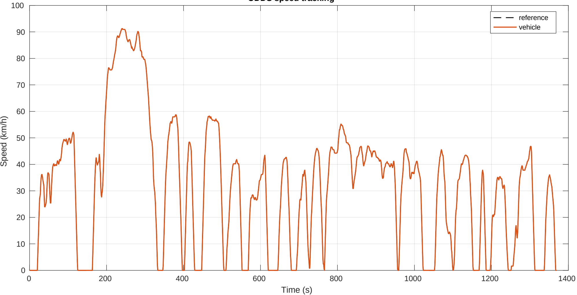
UDDS speed tracking
