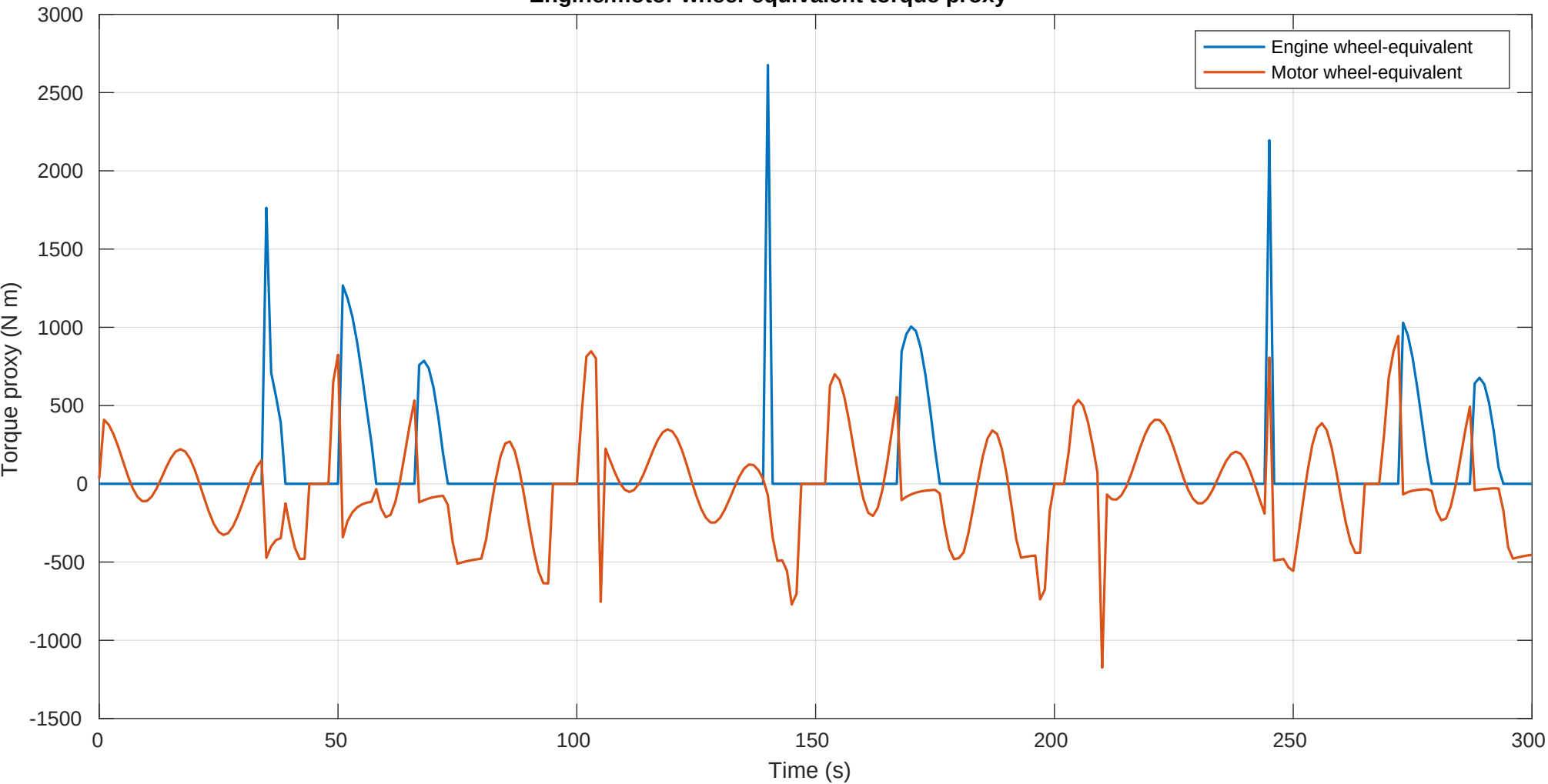
Engine/motor wheel-equivalent torque proxy
