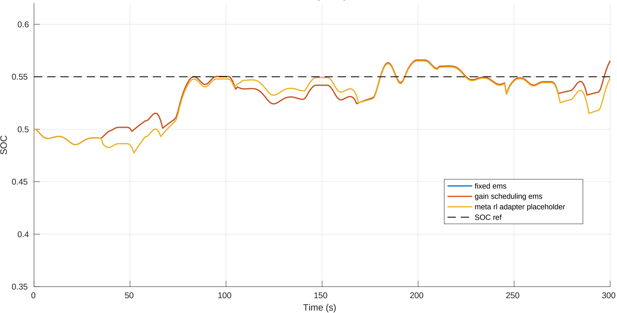
SOC trajectory
