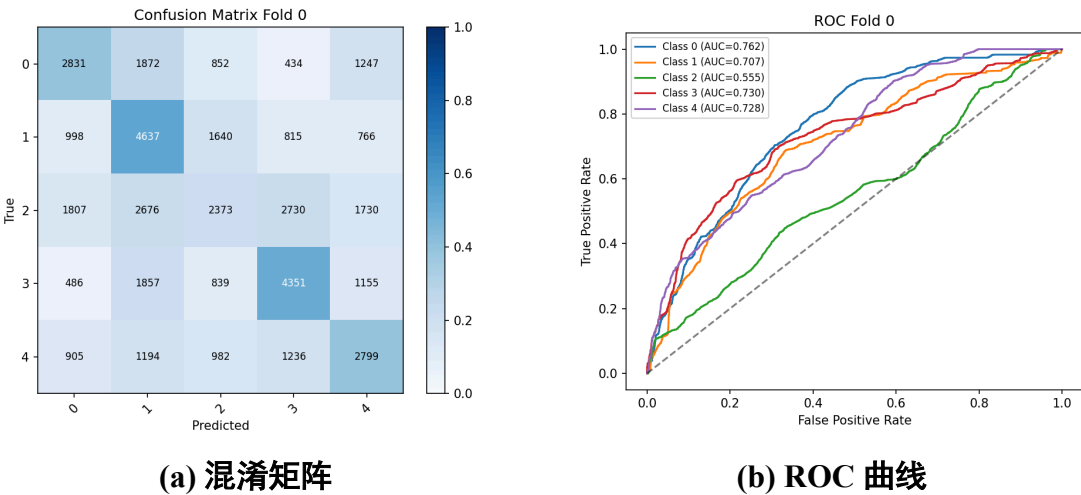
图 4.1 下游评估可视化——基线模型(无 GNN)在 SEED-V 上的 6-fold 交叉验证结果
