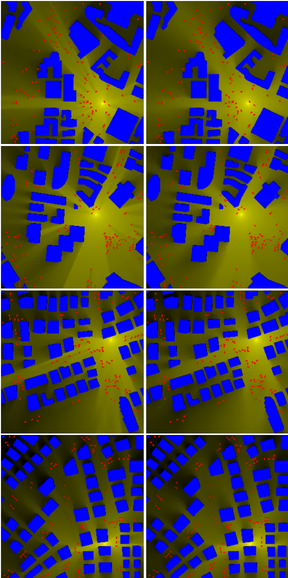
RadioUNet
