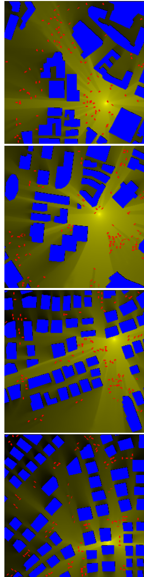
RadioMamba
