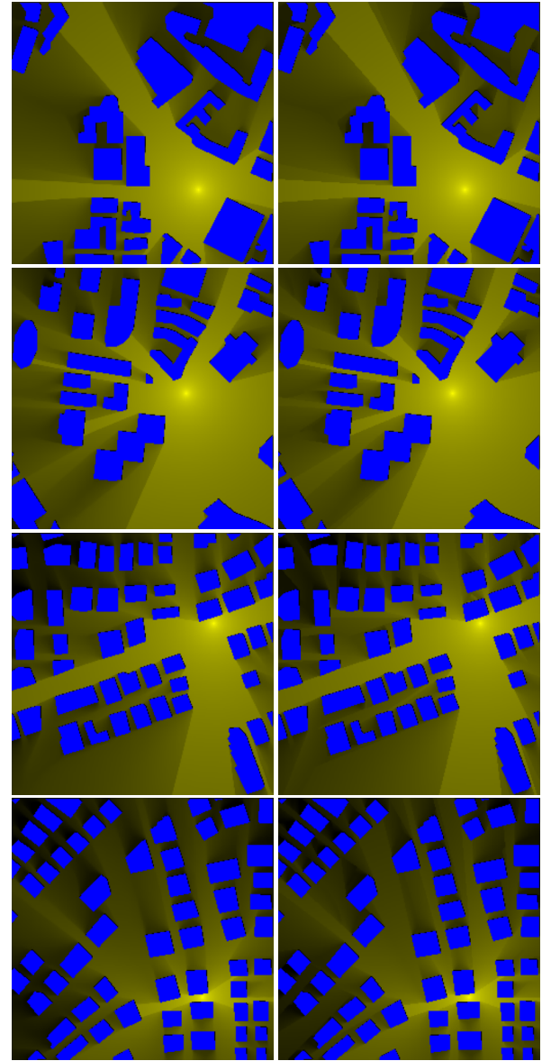
Ours
