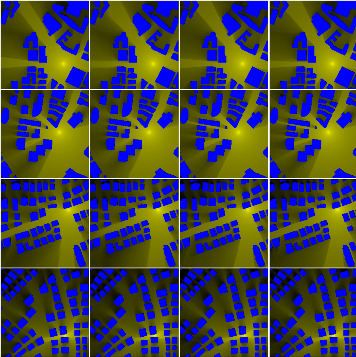
RadioUNet
