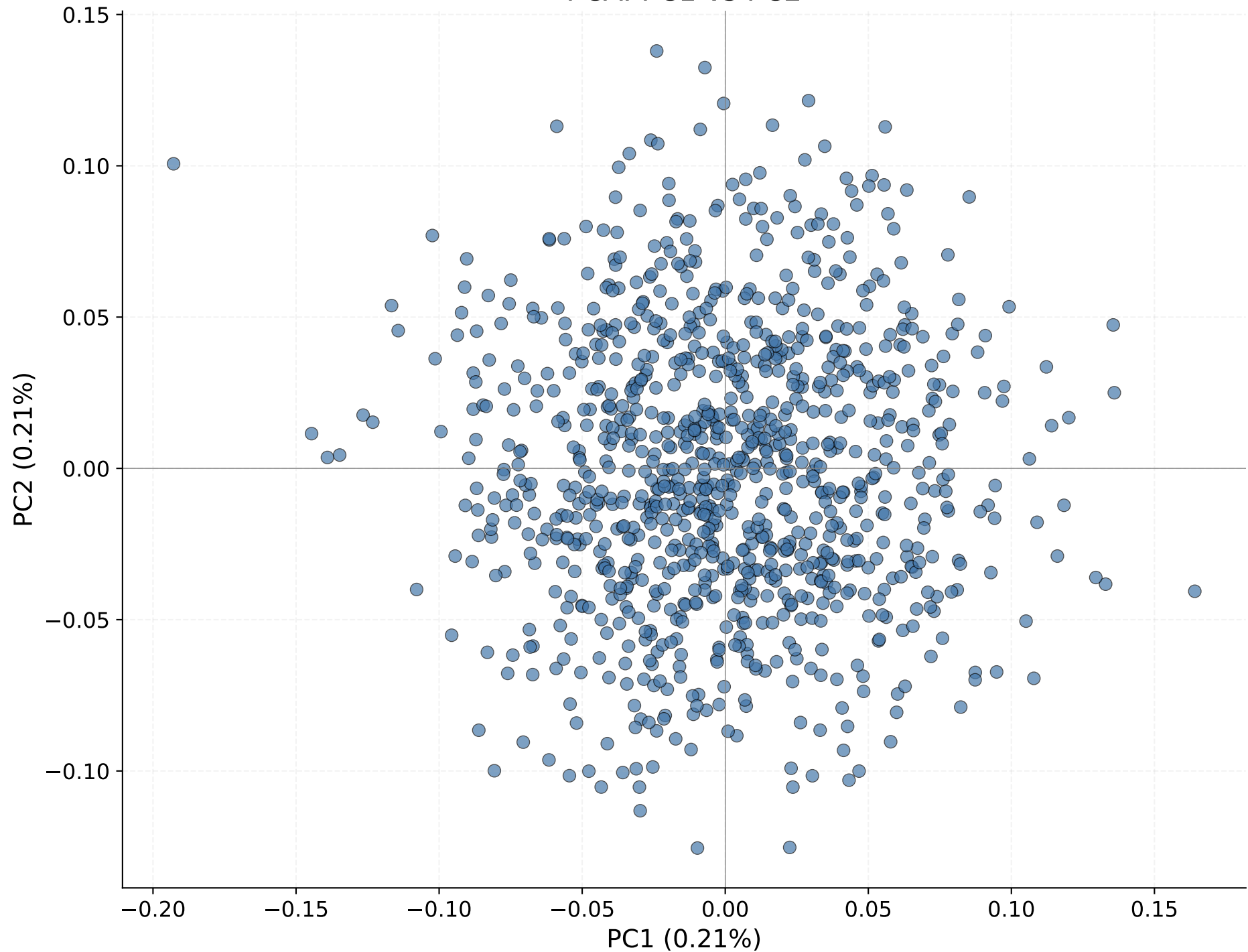
PCA: PC1 vs PC2
