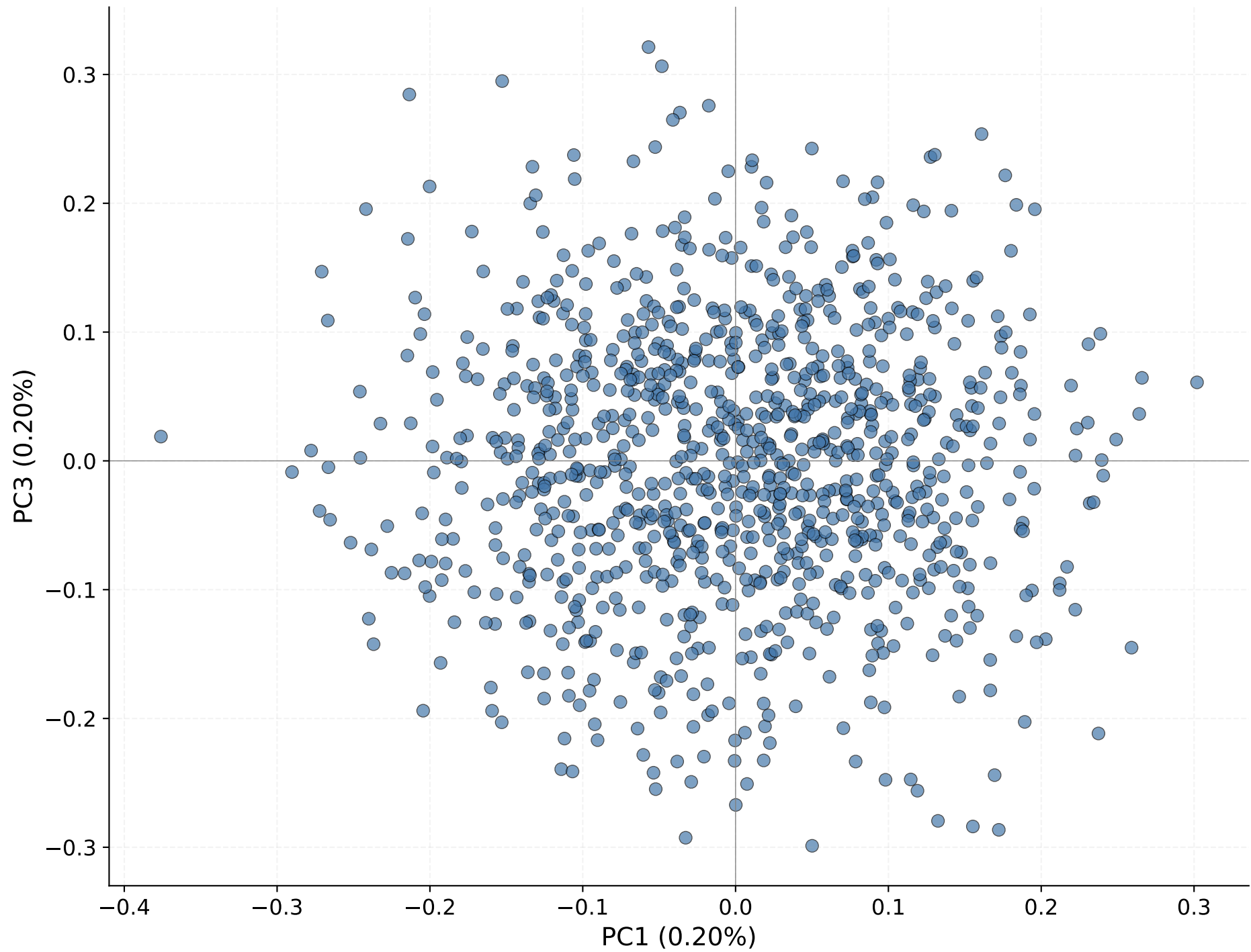
PCA: PC1 vs PC3
