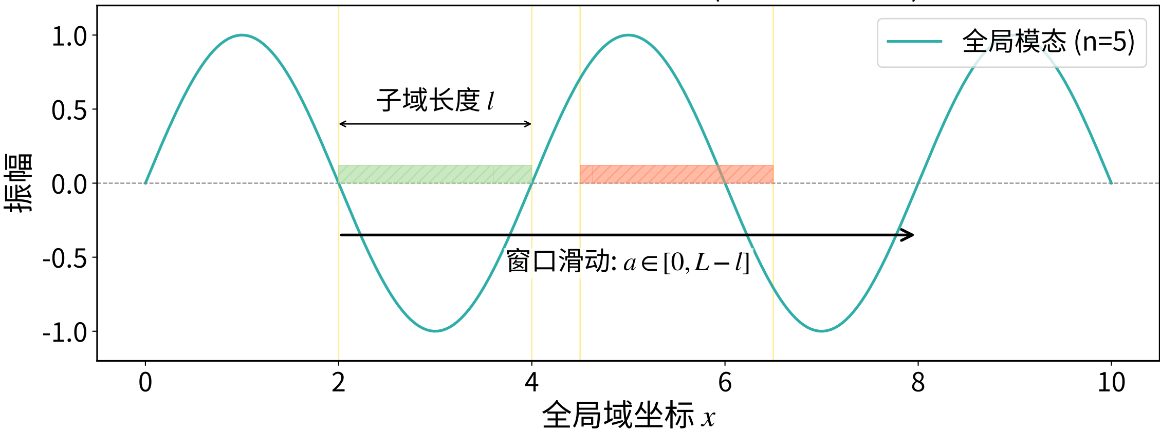
集成误差滑动子结构示意图 (全局模态 n=5 )
