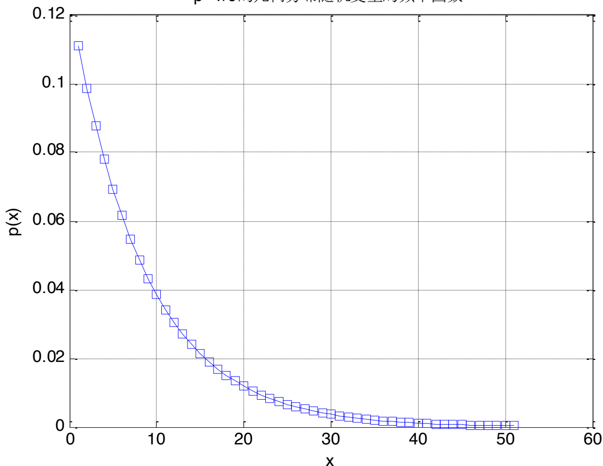
p=1/9 的几何分布随机变量的频率函数
