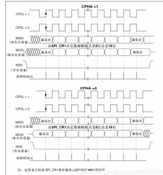
图212 数据时钟时序图
