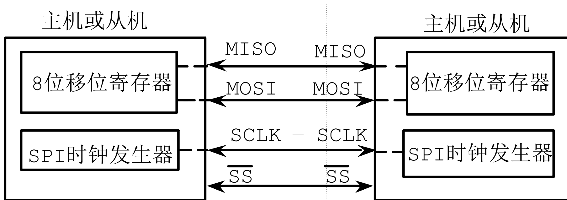
SPI接口的双器件连接方式
