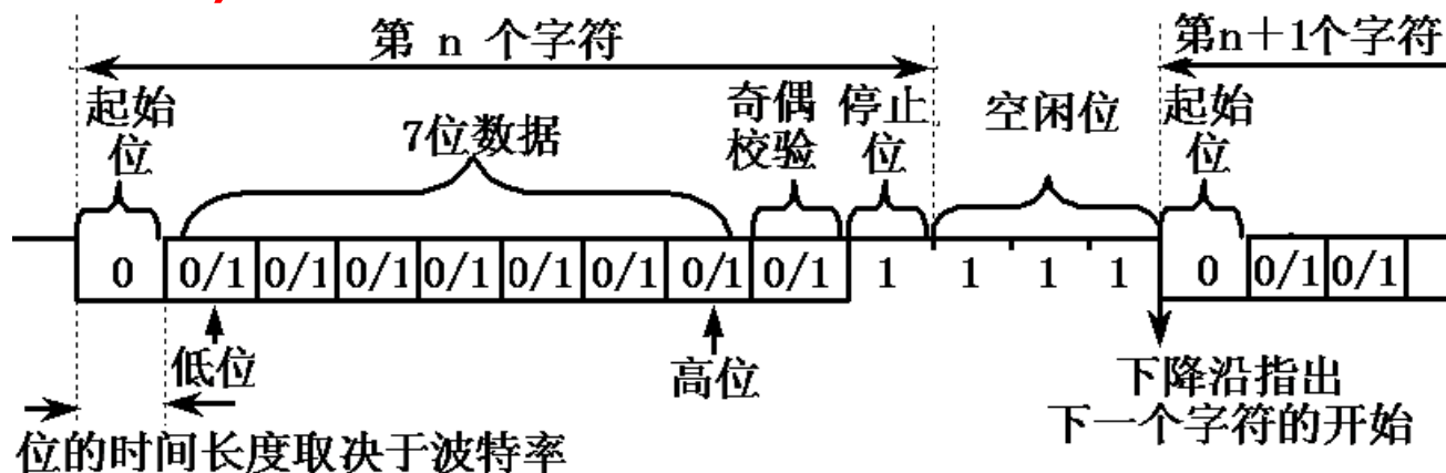
a) 数据字为7位ASCII码时的通信格式
