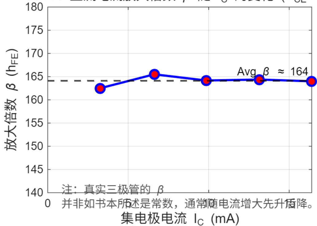
S9013 直流电流放大倍数 \beta 随 I_C 的变化 ( V_{CE}=5V )
