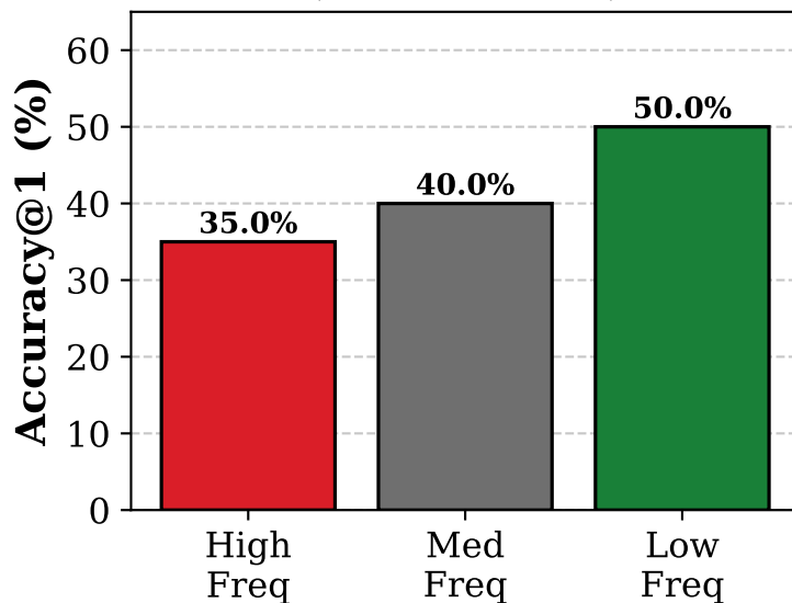
(B) BERT (LAMA Probe)
