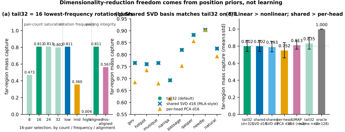
图 4: 降维自由度来自位置先验: (a) tail32 = 16 个完整最低频旋转对 (频率单调、错位配对崩 0.567、16 对饱和); (b) 共享 SVD 基 d=16 在 8/8 样本上追平 tail32; (c) 线性优于非线性、共享优于 per-head——UMAP 仅在 2 样本上评测 (80–167s/层样本的 fit 成本), 成对参照柱给出同 2 样本的 tail32 (0.835 对 0.813)。
