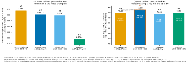
图 5: 质量代理口径与端到端口径的四组合最优配置对照。双口径差异须注明: mass 为 softmax 质量覆盖 (块池 BP=64 、总预算 B_{\text{TOK}}=2048 、16 样本 trace 均值); e2e 为 LongBench hotpotqa+musique 等权均值 (各 n=200 ), K_1=128/K_2=1024 。两 panel 同 x 顺序 (按 mass 降序), 名次标签直观显示反转: mass 冠军 (minmax, minmax) (0.896) 在 e2e 跌至第 3 档 (43.90, 与 (avg, avg) 并列), mass 第 2 的 (minmax, avg) 升为 e2e 冠军 (45.08; hotpotqa 55.44 为全部 13 臂最高, musique 34.71 仅次于 \beta=0.25 臂的 35.57, 该臂平均分 44.86 更低)。柱内白字为各组合 e2e 最优臂的双任务分; 灰色虚线为部署参照臂 ( \gamma=0.125 , 44.59); x 轴第二行为该口径下最优臂的 (\alpha, \beta, \gamma) ; (cluster, cluster) 无 e2e 实现路径仅 mass 数据, 如实排除。
