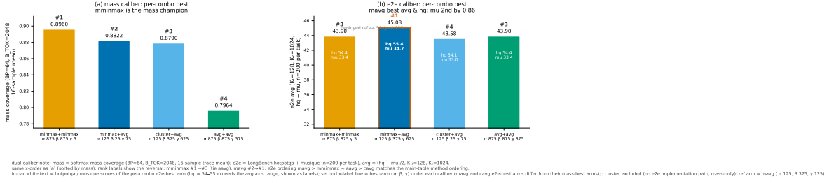
图 5: 质量代理口径与端到端口径的四组合最优配置对照。双口径差异须注明: mass 为 softmax 质量覆盖(块池 BP=64 、总预算 B_{\text{TOK}}=2048 、16 样本 trace 均值); e2e 为 LongBench hotpotqa+musique 等权均值 (各 n=200 ), K_1=128/K_2=1024 。两 panel 同 x 顺序 (按 mass 降序), 名次标签直观显示反转: mass 冠军 (minmax, minmax) (0.896) 在 e2e 跌至第 3 档 (43.90, 与 (avg, avg) 并列), mass 第 2 的 (minmax, avg) 升为 e2e 冠军 (45.08; hotpotqa 55.44 为全部 13 臂最高, musique 34.71 仅次于 \beta=0.25 臂的 35.57, 该臂平均分 44.86 更低)。柱内白字为各组合 e2e 最优臂的双任务分; 灰色虚线为部署参照臂 ( \gamma=0.125 , 44.59); x 轴第二行为该口径下最优臂的 (\alpha, \beta, \gamma) ; (cluster, cluster) 无 e2e 实现路径仅 mass 数据, 如实排除。
