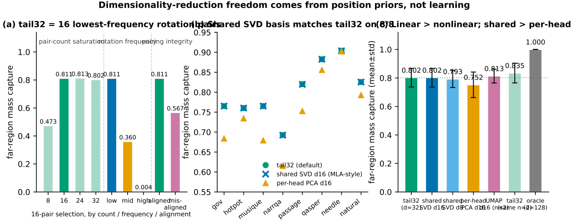
图 4: 降维自由度来自位置先验：(a) tail32 = 16 个完整最低频旋转对（频率单调、错位配对崩 0.567、16 对饱和）；(b) 共享 SVD 基 d=16 在 8/8 样本上追平 tail32；(c) 线性优于非线性、共享优于 per-head——UMAP 仅在 2 样本上评测（80–167s/层样本的 fit 成本），成对参照柱给出同 2 样本的 tail32（0.835 对 0.813）。
