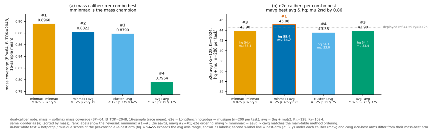
图 5: 质量代理口径与端到端口径的四组合最优配置对照。双口径差异须注明: mass 为 softmax 质量覆盖(块池 BP=64 、总预算 B_{\text{TOK}}=2048 、16 样本 trace 均值); e2e 为 LongBench hotpotqa+musique 等权均值 (各 n=200 ), K_1=128/K_2=1024 。两 panel 同 x 顺序 (按 mass 降序), 名次标签直观显示反转: mass 冠军 (minmax, minmax) (0.896) 在 e2e 跌至第 3 档 (43.90, 与 (avg, avg) 并列), mass 第 2 的 (minmax, avg) 升为 e2e 冠军 (45.08; hotpotqa 55.44 为全部 13 臂最高, musique 34.71 仅次于 \beta=0.25 臂的 35.57, 该臂平均分 44.86 更低)。柱内白字为各组合 e2e 最优臂的双任务分; 灰色虚线为部署参照臂 ( \gamma=0.125 , 44.59); x 轴第二行为该口径下最优臂的 (\alpha, \beta, \gamma) ; (cluster, cluster) 无 e2e 实现路径仅 mass 数据, 如实排除。
