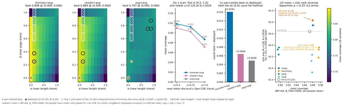
图 2: 预算参数面 ( \alpha/\beta/\gamma 扫描): \beta 0.25–0.75 平坦、 \alpha 单调至边界, per-task/per-layer oracle 上限 +0.08/+0.0008——参数不需精调本身构成部署优势; panel (d) 为 13 个端到端配置臂的离线质量代理对端到端精度散点——两口径秩相关弱 (排序反转), 配置选举只认端到端实测 (详见消融节)。
