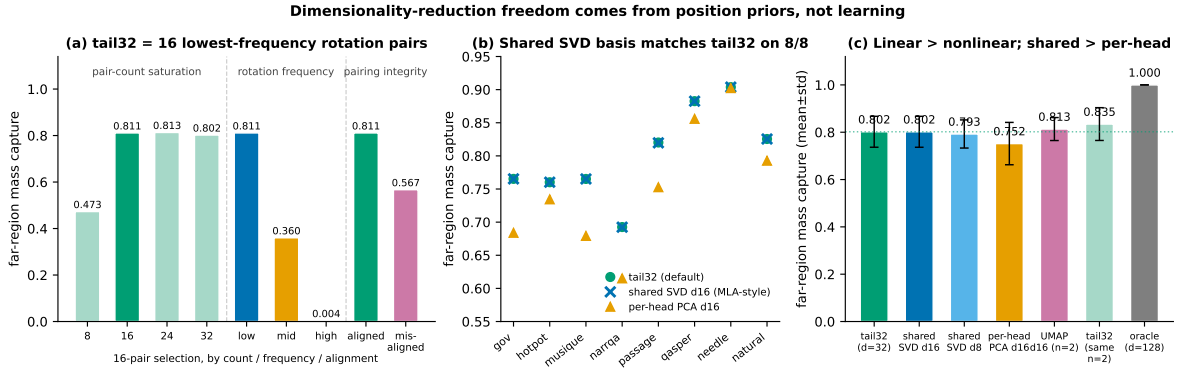
图 4: 降维自由度来自位置先验：(a) tail32 = 16 个完整最低频旋转对（频率单调、错位配对崩 0.567、16 对饱和）；(b) 共享 SVD 基 d=16 在 8/8 样本上追平 tail32；(c) 线性优于非线性、共享优于 per-head——UMAP 仅在 2 样本上评测（80–167s/层样本的 fit 成本），成对参照柱给出同 2 样本的 tail32（0.835 对 0.813）。
