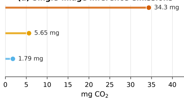
(d) Single-image inference emissions
