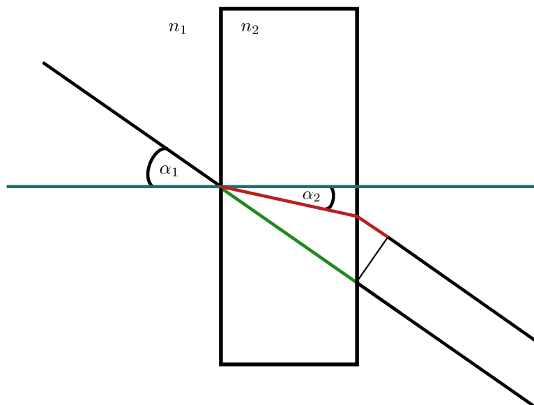
Figure 2.1: We- gun- ter- schied bei Strahlen- gang durch Glas- plättchen.
