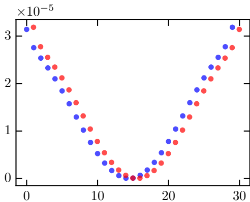
phonon direction y
