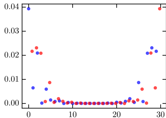
phonon direction y
