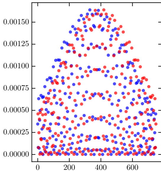
phonon direction y
