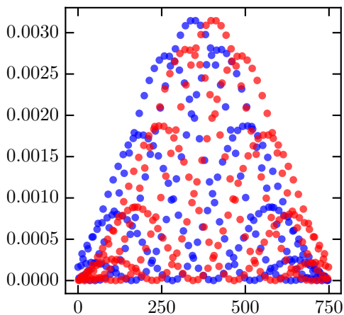
phonon direction y
