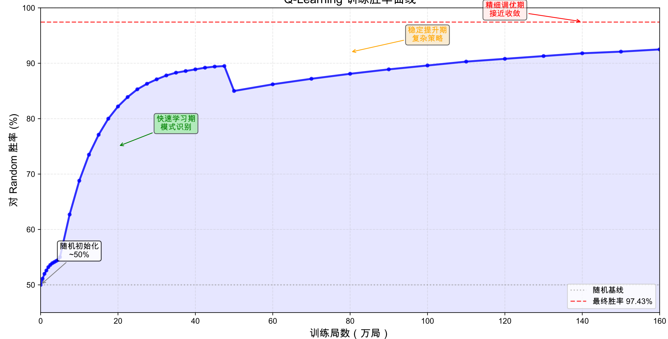
Q 表收敛曲线
