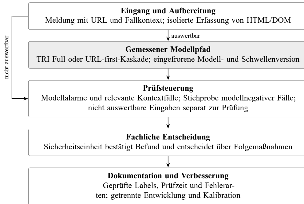
Abbildung 7.1.: Konzipierte Einbettung der Webseitenklassifikation in die fachliche Fallprüfung. Nur der grau hinterlegte Modellpfad wurde experimentell untersucht.
