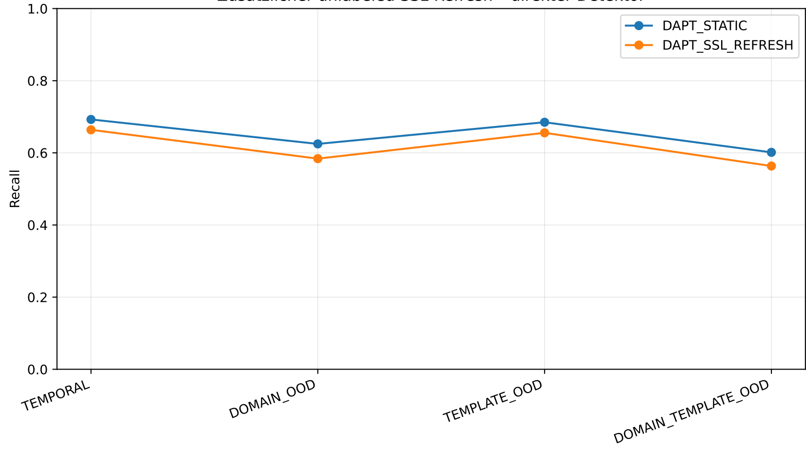
Zusätzlicher unlabeled SSL-Refresh - direkter Detektor
