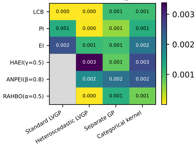
piston (final regret, n_rep=10)
