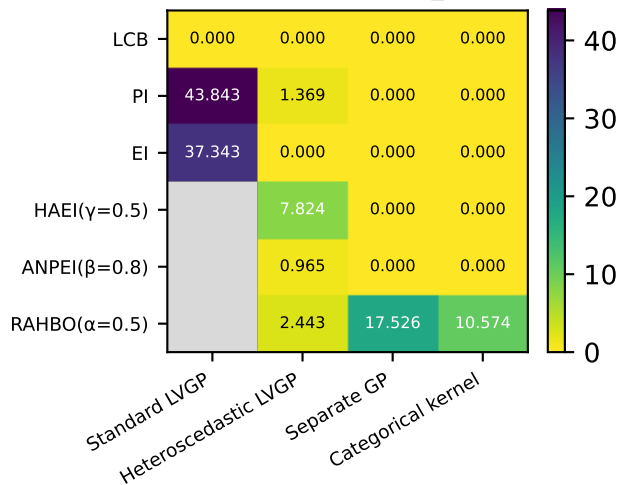
golinski (final regret, n_rep=10)
