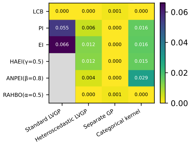
otl_circuit (final regret, n_rep=10)
