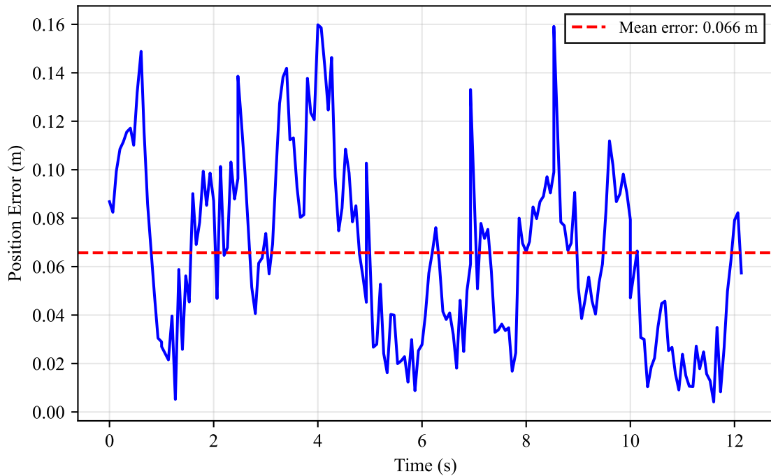
Tracking Error (max: 0.160 m, min: 0.004 m)
