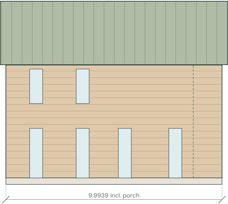
RIGHT ELEVATION
