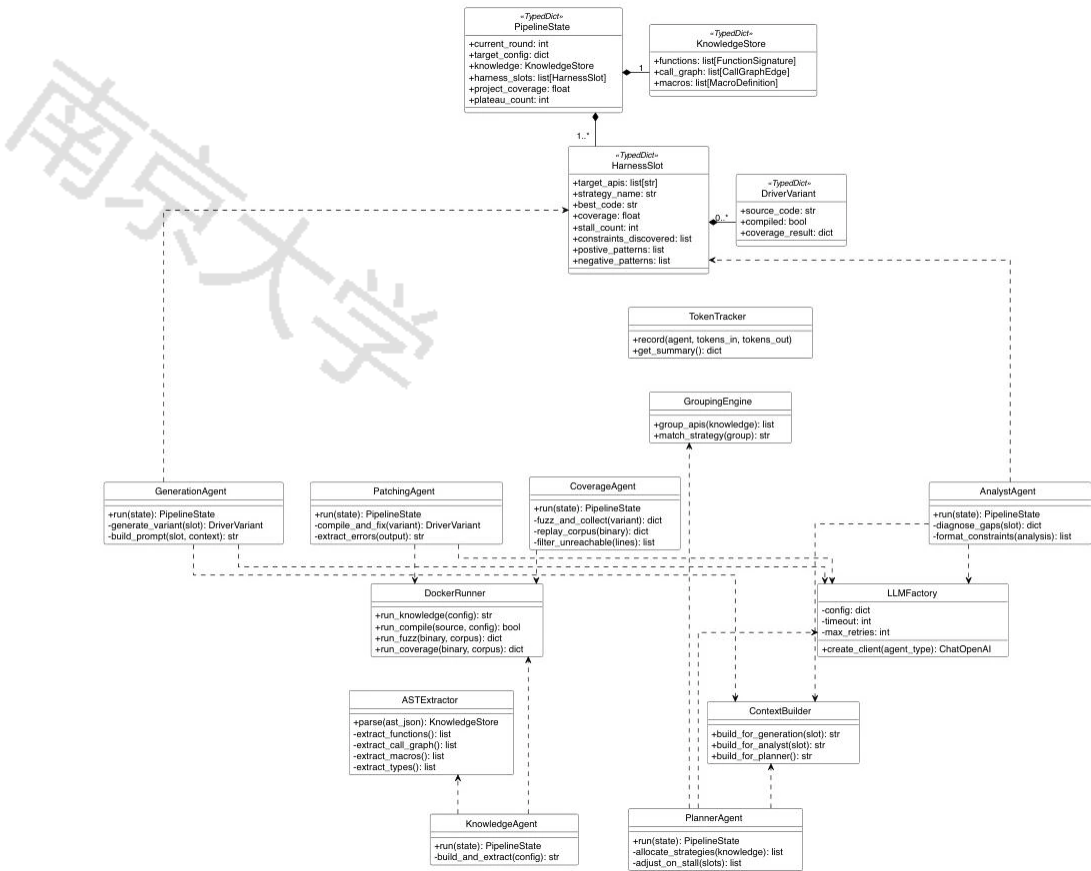
图3-4 MAGIC4FDG系统逻辑视图
