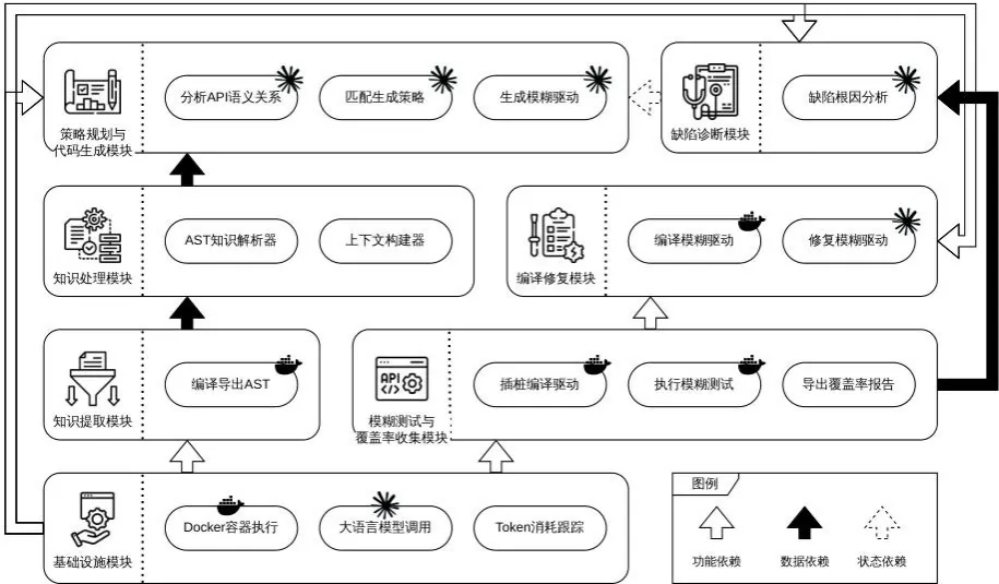
图3-3 MAGIC4FDG 系统整体架构图
