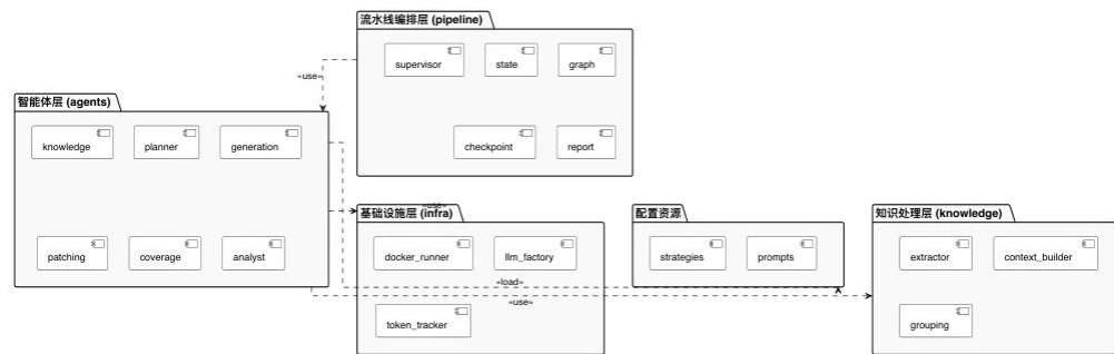
图3-5 MAGIC4FDG系统开发视图
