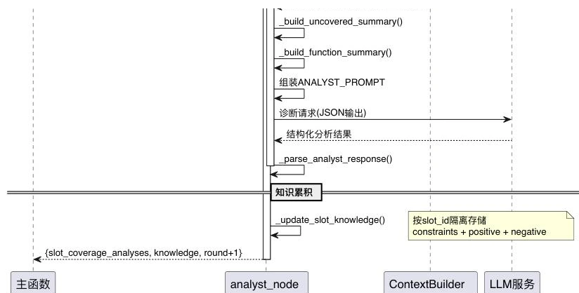
图 4-24 缺口诊断模块详细设计顺序图
