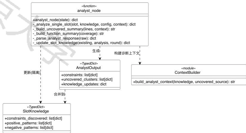
图4-23 缺口诊断模块详细设计类图
