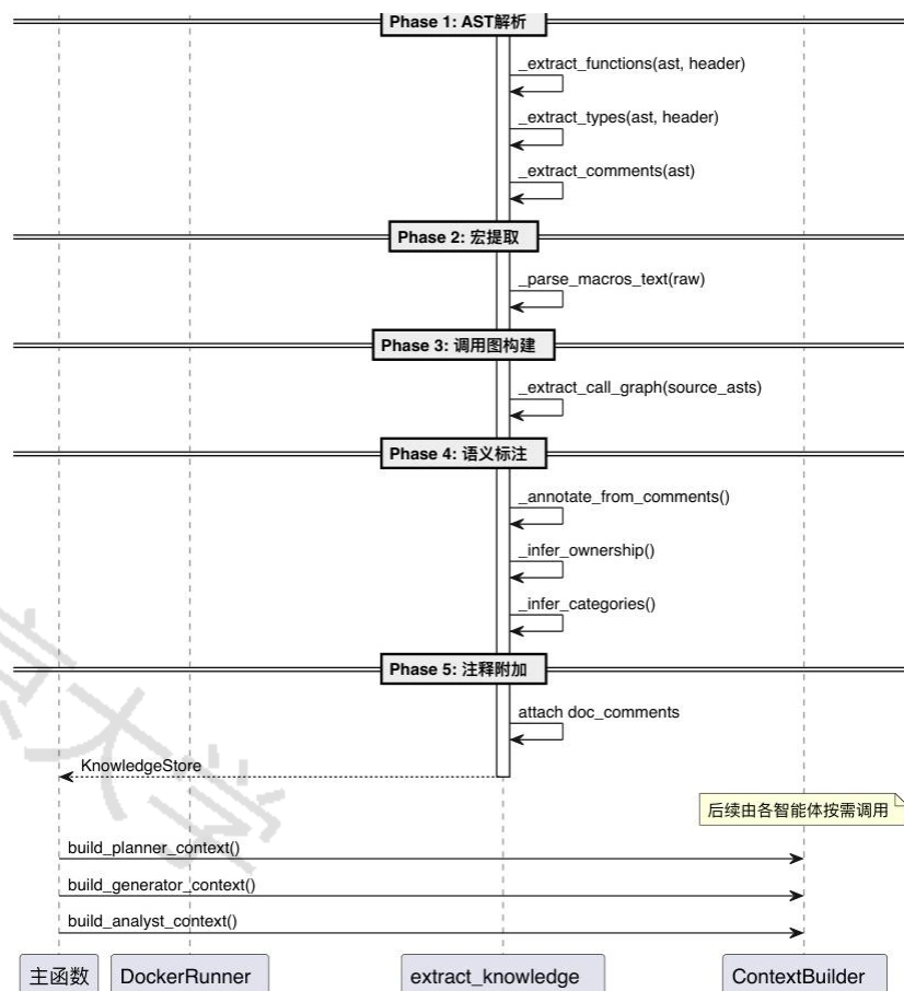
图4-2 知识提取模块详细设计顺序图
