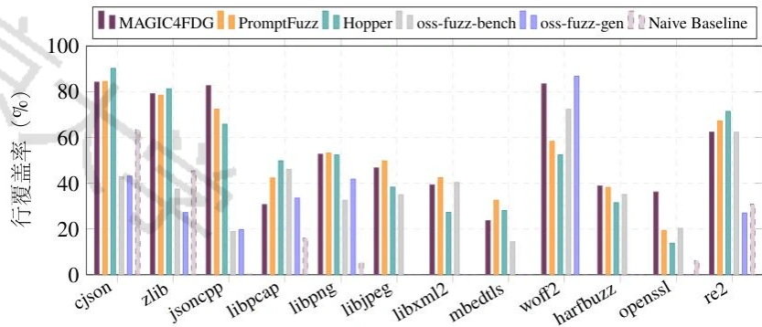
图5-1 12个目标库行覆盖率对比图
