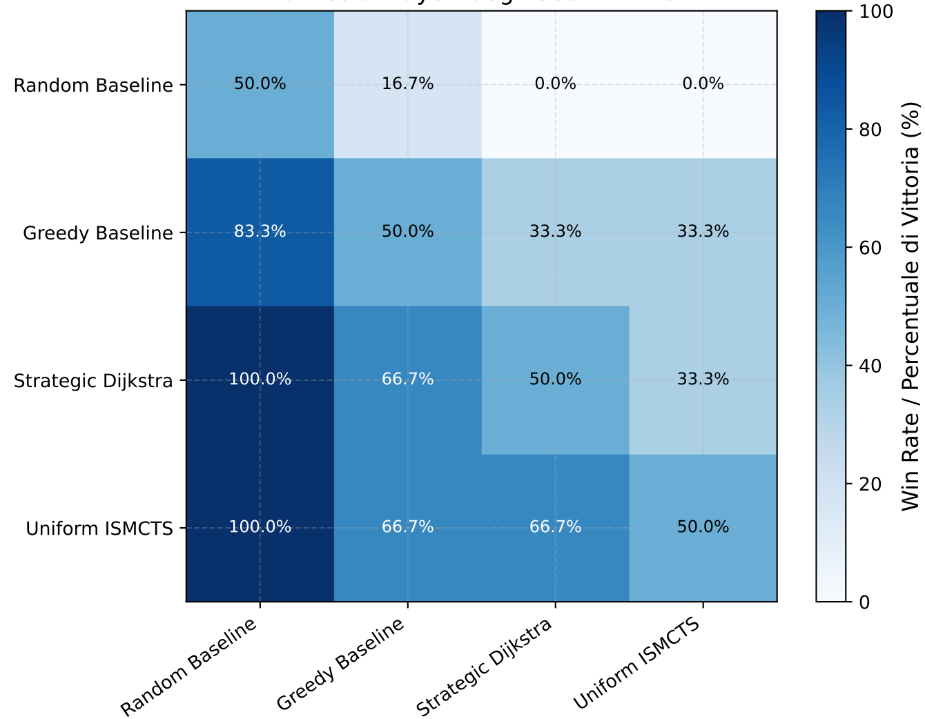
(a) Cross-Matchup Payoff Matrix Matrice di Payoff degli Scontri Diretti
