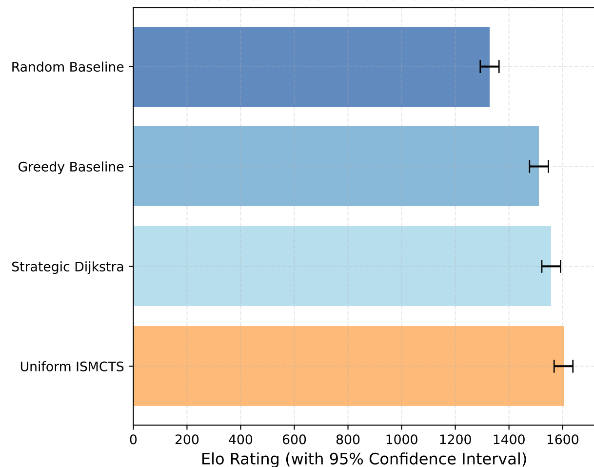
(b) Estimated Elo Ranking Classifica Elo con Intervallo di Confidenza
