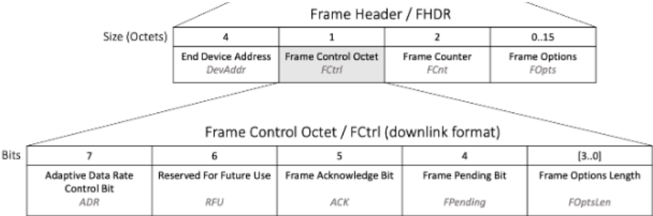
Figura 2 – Campos contidos em Frame Header em Downlink
