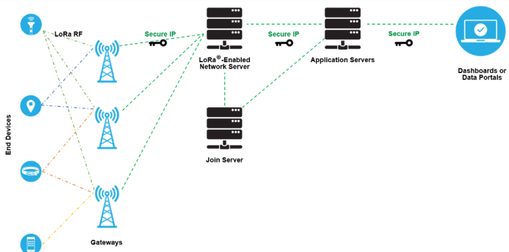
Figura 4 – Implementação Típica de Rede LoRaWan
