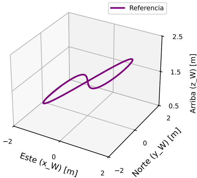
c) Familia LISSAJOUS (Aceleración en 3 Ejes)
