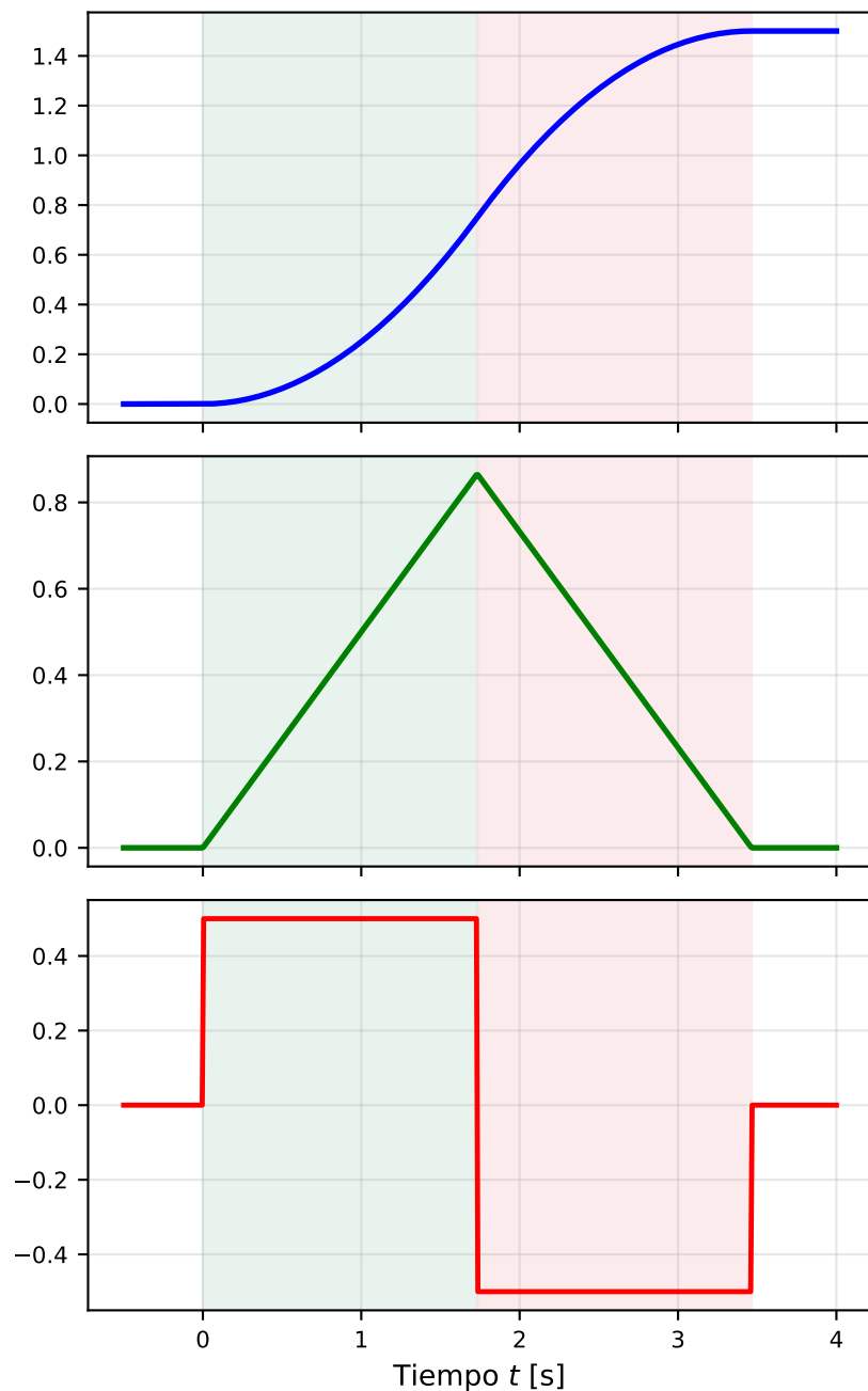
Perfil Triangular ( L = 1.5 m)
