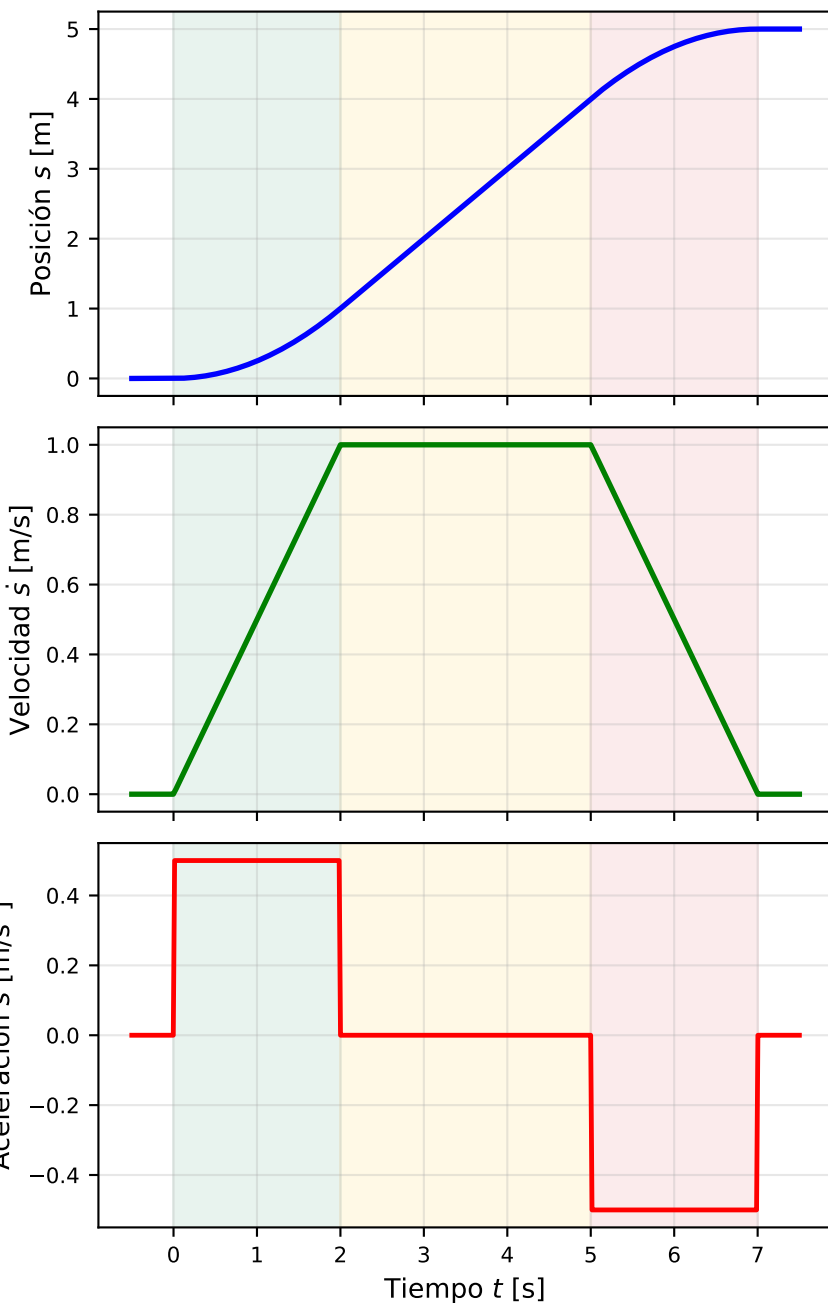
Perfil Trapezoidal ( L = 5.0 m)
