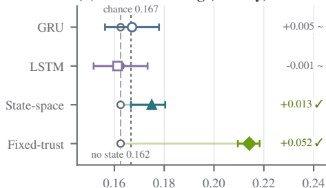
(d) PushT · binding (six-way)
