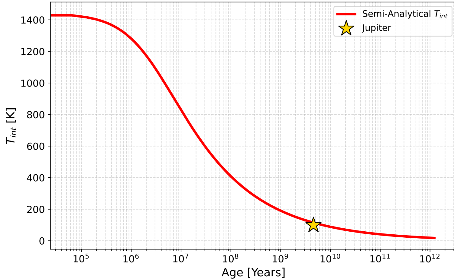
Thermal Evolution (Numerical Int.)
