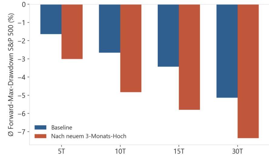
VIX neues „3-Monats-Hoch“
