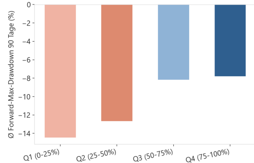
Marktbreite in Quartilen
