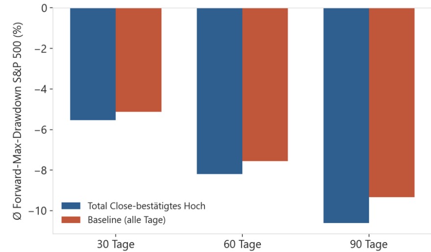
Bestätigung von Extrem-Hochs
