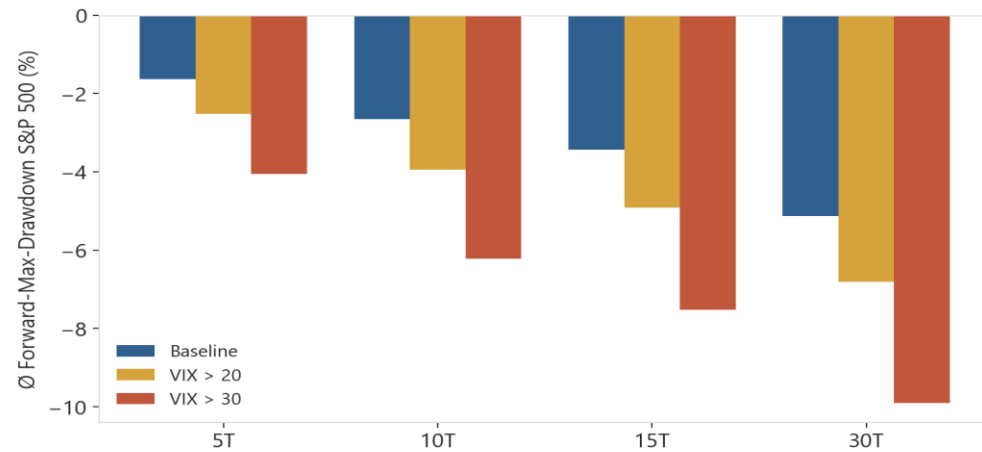
VIX je Ausgangsniveau
