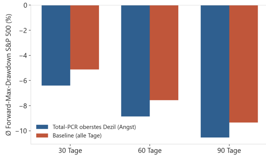
PCR innerhalb oberstem Dezil
