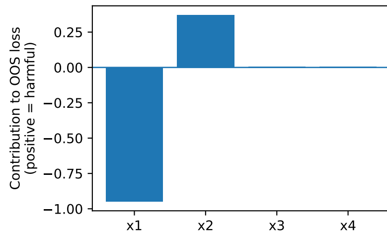
OLS: GPBSV (MSE)
