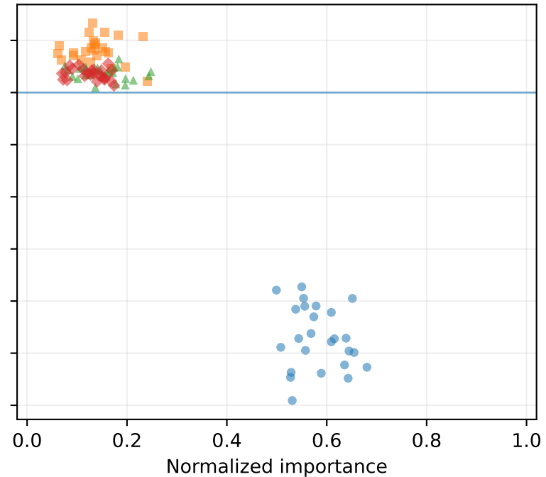
PDP-VI
