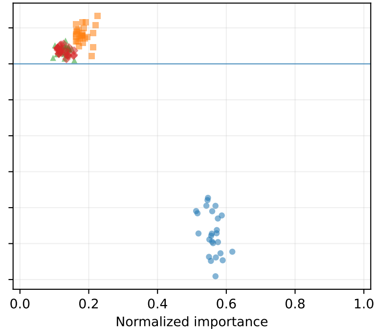
TS-Shapley-VI
