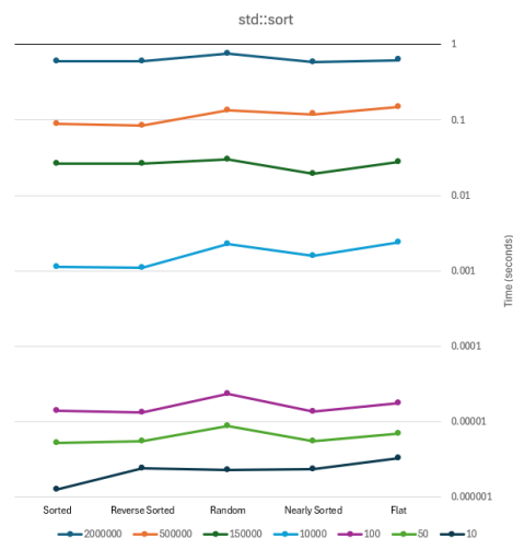
Figure 5. Rezultatele testării std::sort .
