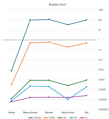
Figure 1. Rezultatele testării Bubble Sort.
